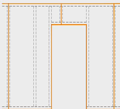
Afbeelding 3.5: Deuropening met voegopvulling
