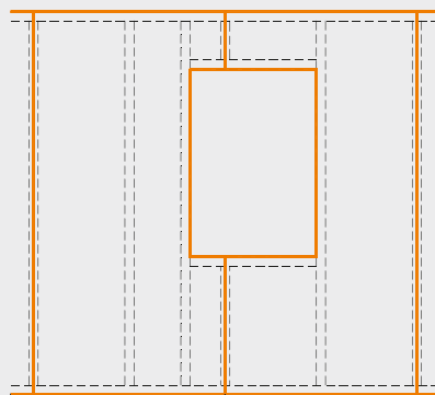
Afbeelding 3.6: Raamopening met voegopvulling
